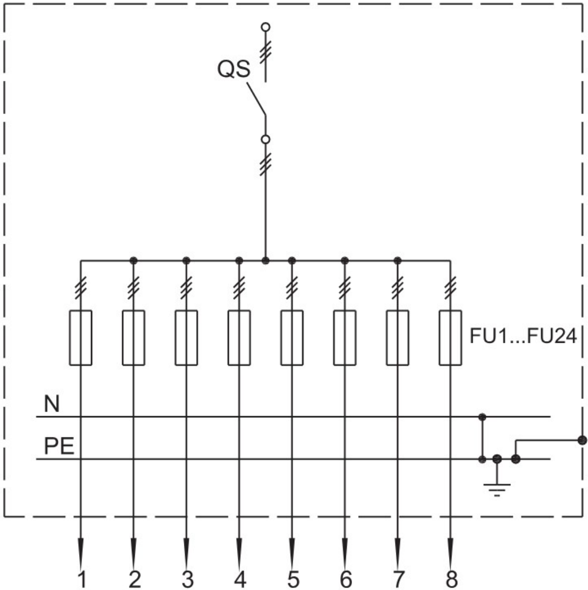
Схема электрическая принципиальная, Щит Распределительный, ШР-11-73505, 400А.
